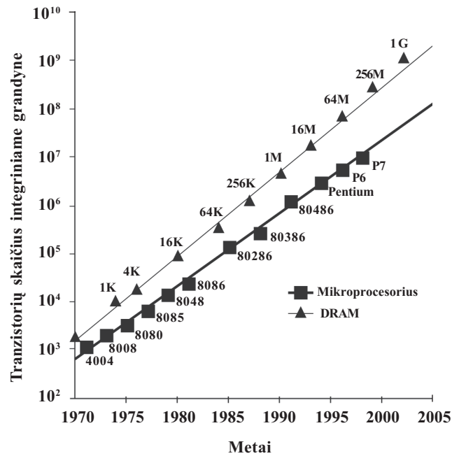
2.7 pav. Tranzistorių skaičiaus integriniame grandyne ir jo atminties (DRAM) talpos didėjimas
